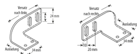
Versetzter Befestigungswinkel
