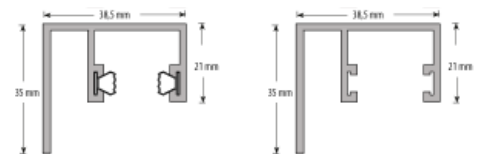
Führungsschiene unten mit L-Lappen (mit / ohne Gleitkeder)
