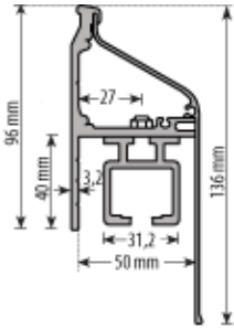
Profilkit Schiebeläden 1-spurig
