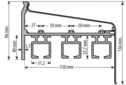
Profilkit Schiebeläden 3-spurig
