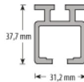
Obere Führungsschiene (einzeln)
