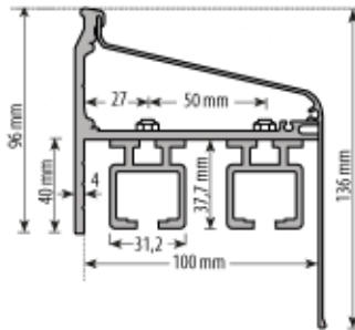
Profilkit Schiebeläden 2-spurig
